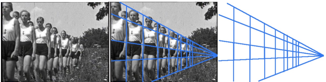
Abbildung 2: Ordnungsbildung Marschieren
